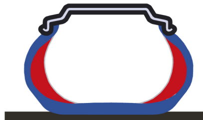
opona RunOnFlat
